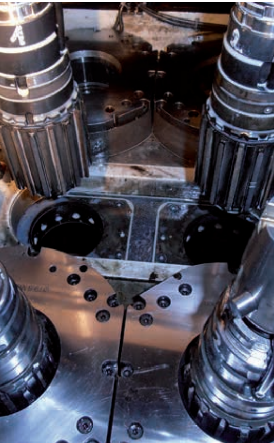
Werkzeugwechsler nach Umbau
