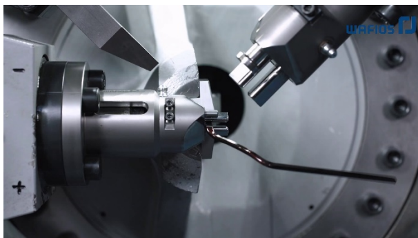
BU: Hairpin-Prototypen Herstellung auf WAFIOS FMU-E
