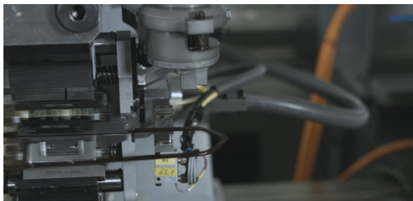
BU: Hairpin Biegeprozess auf WAFIOS SpeedFormer
