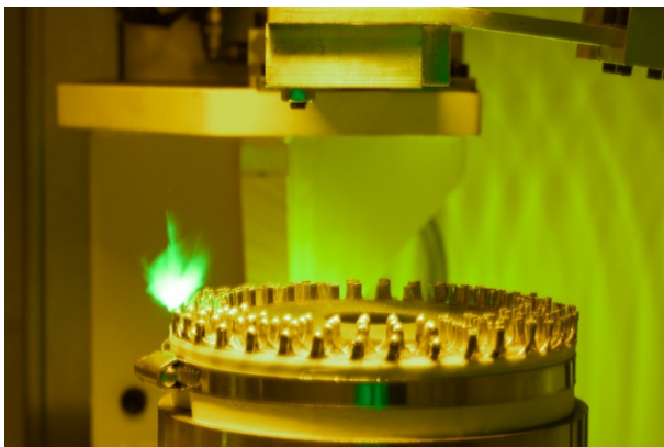
BU: Laserschweißen eines Stators.
