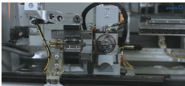
BU: Hairpin Biegeprozess auf WAFIOS SpeedFormer
